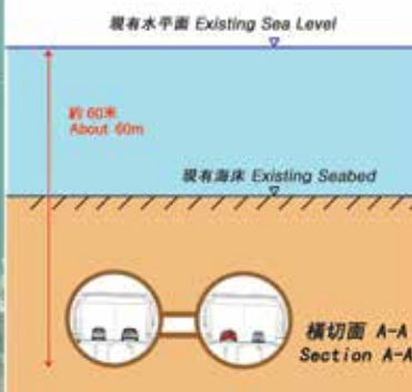
屯門至赤鱗角連接路由大嶼山經港珠澳大橋人工島，以過海隧方式連接屯門。
